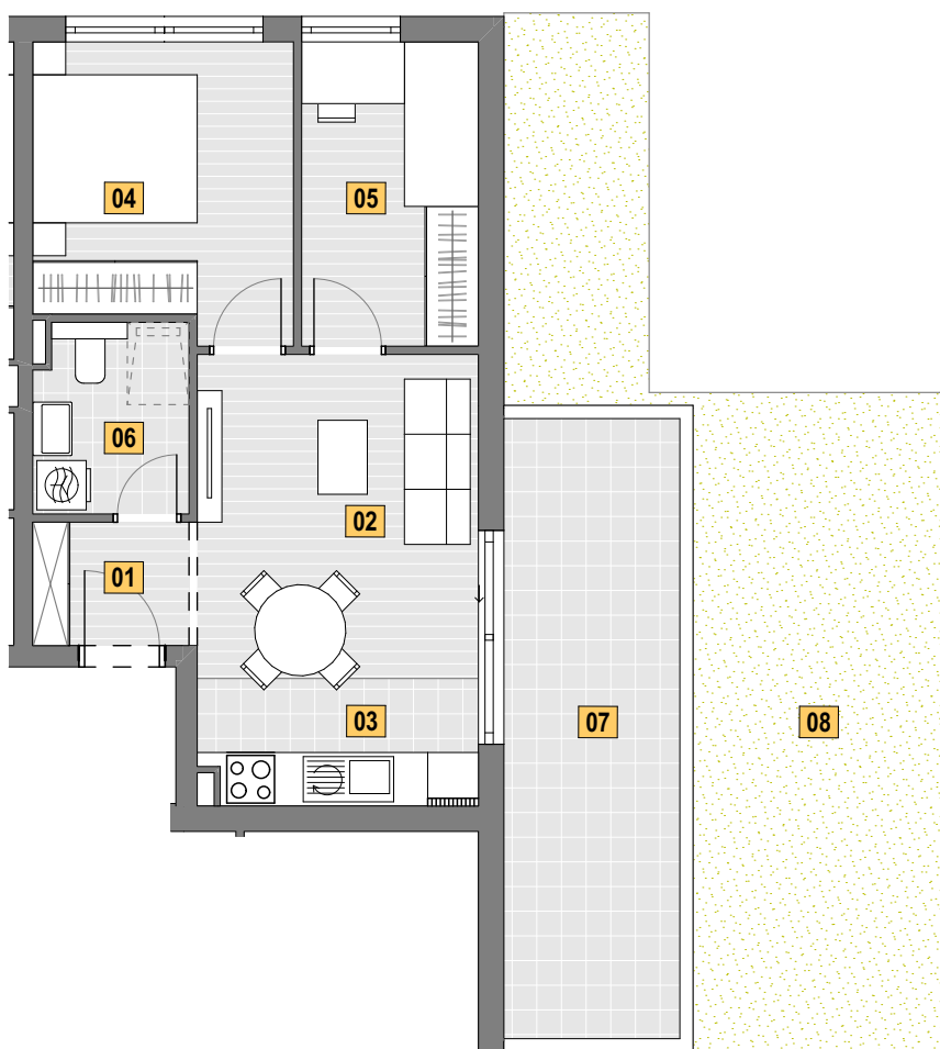
TLOCRT STANA
