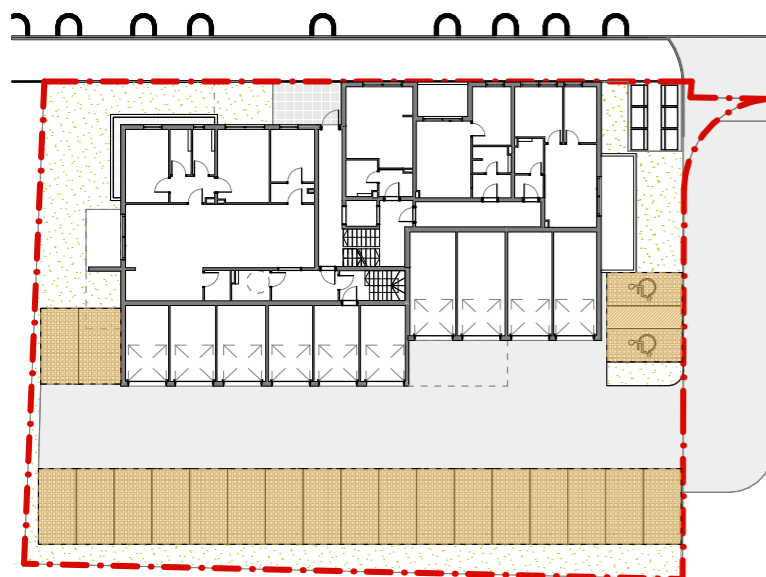
TLOCRT PRIZEMLJA
