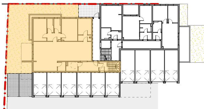
TLOCRT PRIZEMLJA
