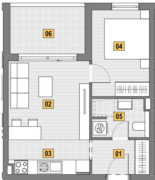
TLOCRT STANA
