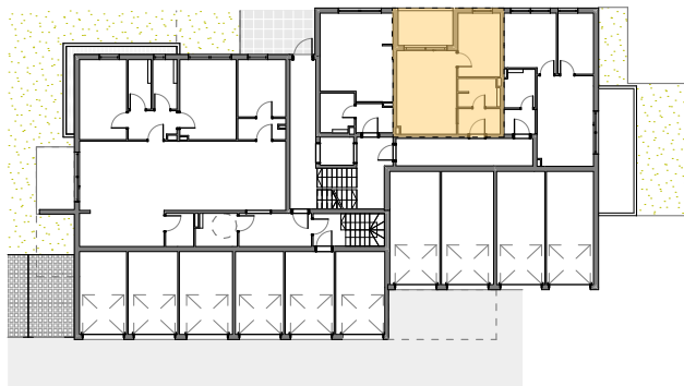
TLOCRT PRIZEMLJA
