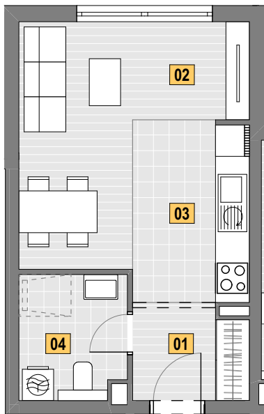
TLOCRT STANA
